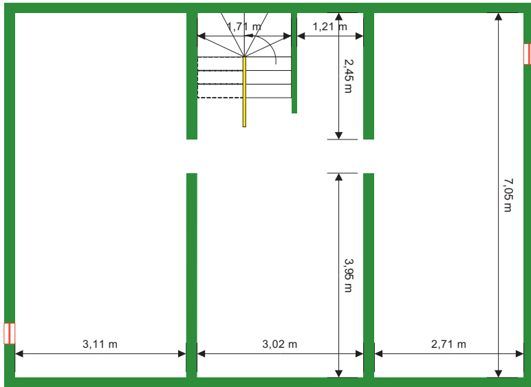
Sous-sol
