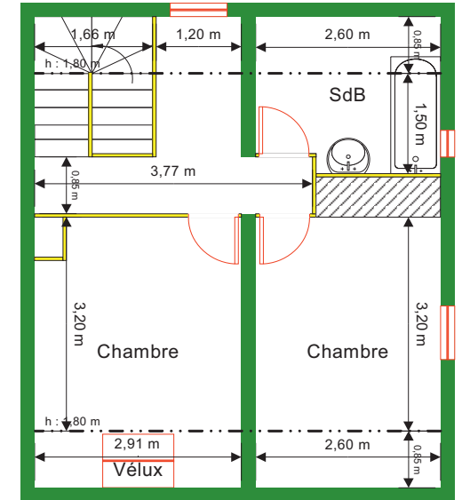
1 er étage
